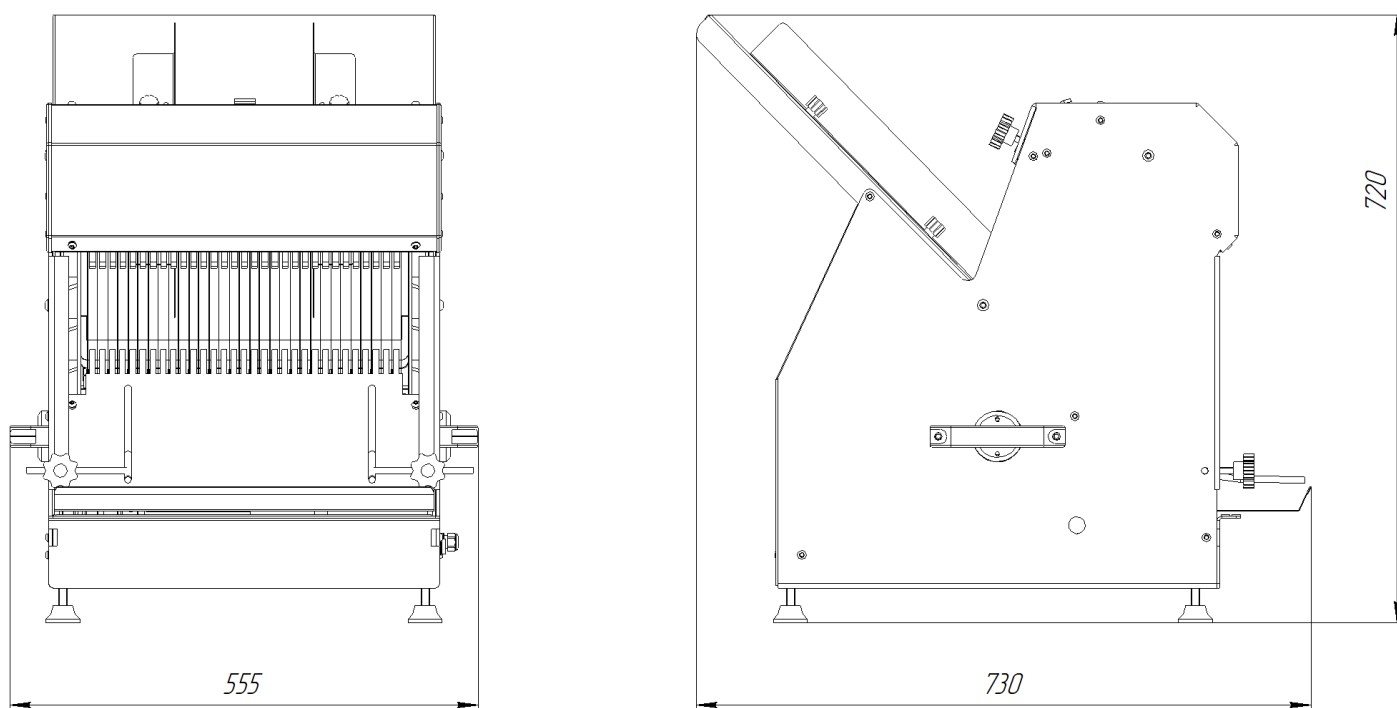
Рис.1. Габаритные размеры.
